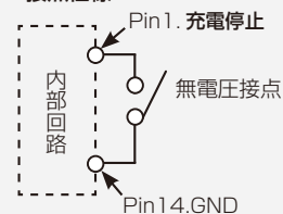
B 接点仕様
