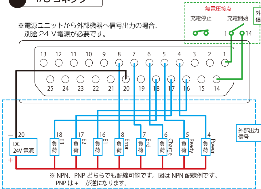
コネクタ（ケーブル配線側）の嵌合面
