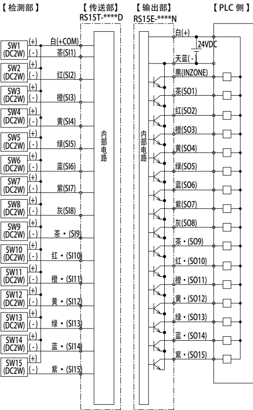
C031 直流 2 线式规格 信号传送通道数：15 路 环形 RS15T-R01D / RS15E-R02_ , RS15T-R03D / RS15E-R03_
