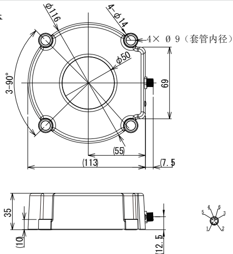
输出头
