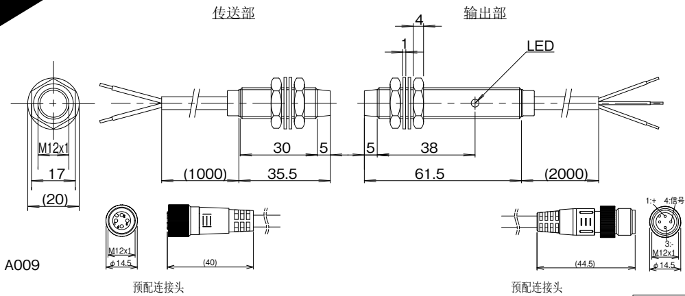
连线图 C012/P. 102
