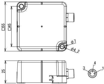
传送头
