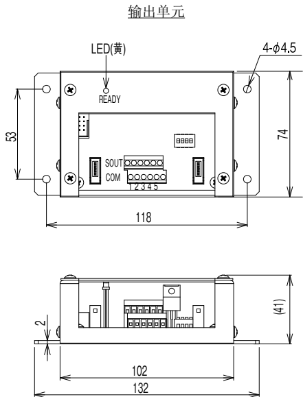
A053 连线图 请参阅《产品手册》。
