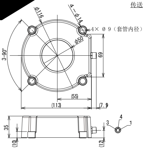
传送头
