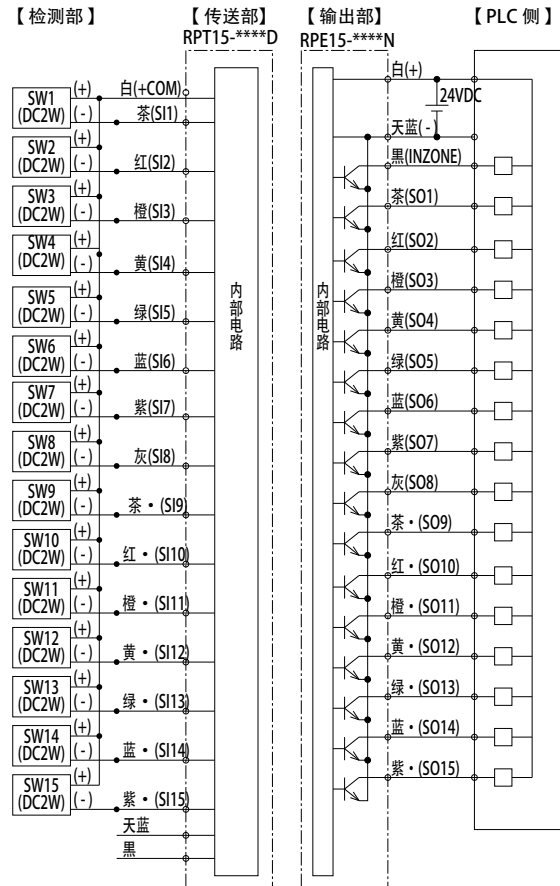
C011 直流 2 线式规格 信号传送通道数：15 路 RPT15-3005D / RPE15-3000_
