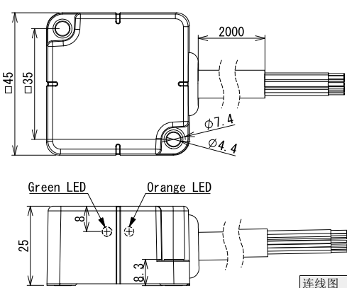
输出部
