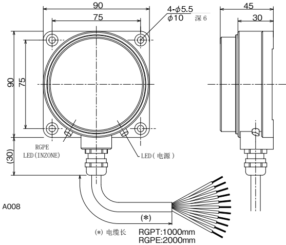
传送部、输出部尺寸图 (共通)
